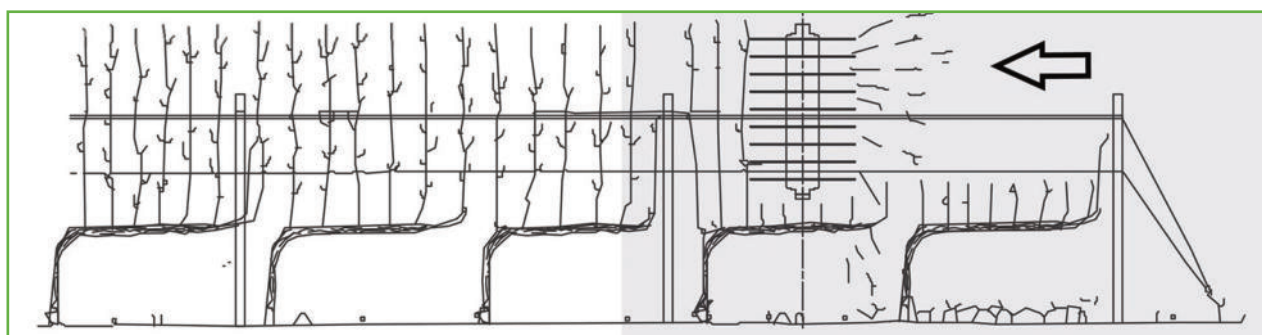
Схема роботи машини для попереднього зимового обрізання
